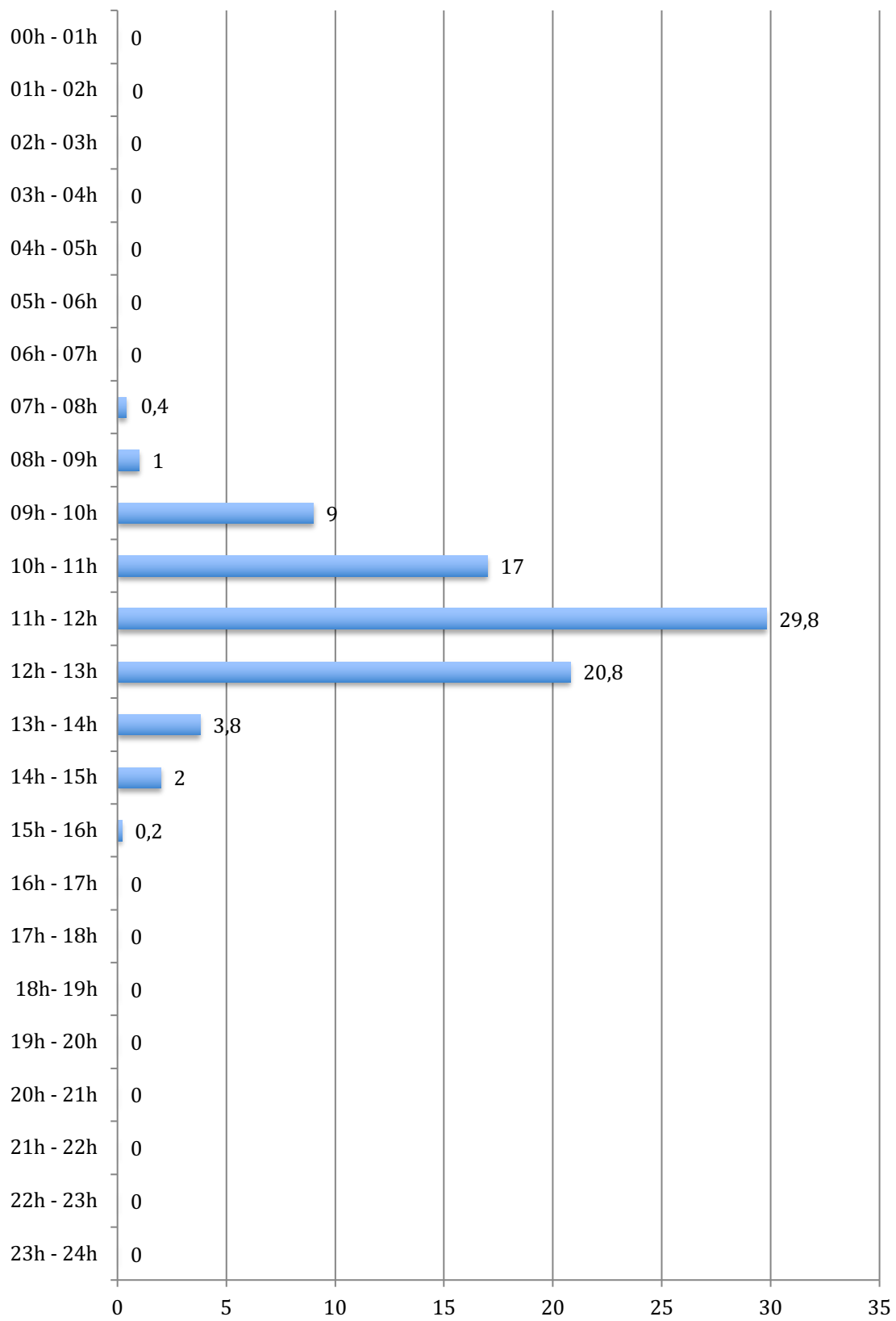
Cantidades de lluvia registradas por horas en BENIGÀNIM el día 16/05/20 (en l/m²)
