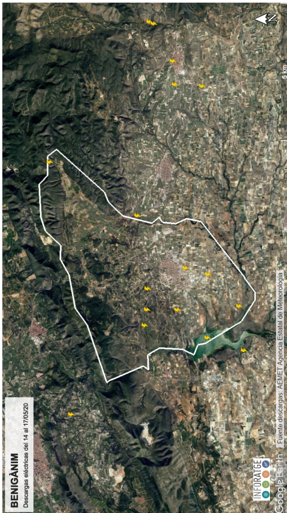
Geolocalización de las descargas eléctricas ~ nube-tierra registradas en el término municipal de BENIGÀNIM y alrededores entre el 14 y el 17/05/20 Fuente descargas: AEMET Agencia Estatal de Meteorología
